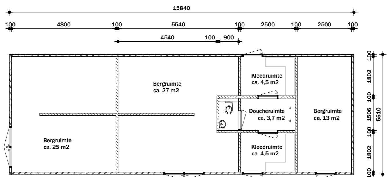
Plattegrond nieuw
